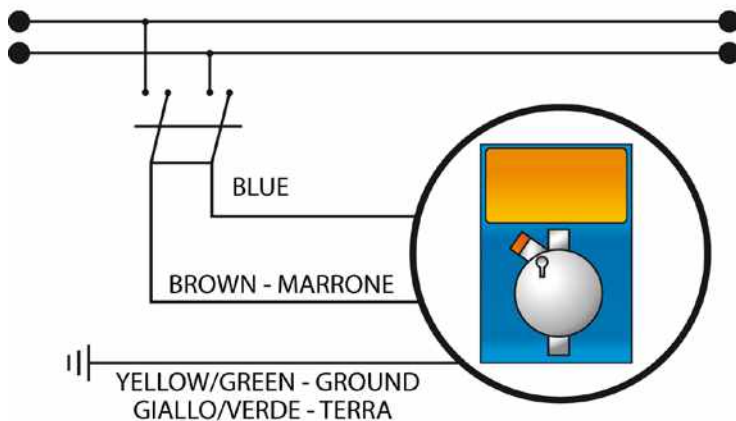
Fig.3 - Branchement électrique
