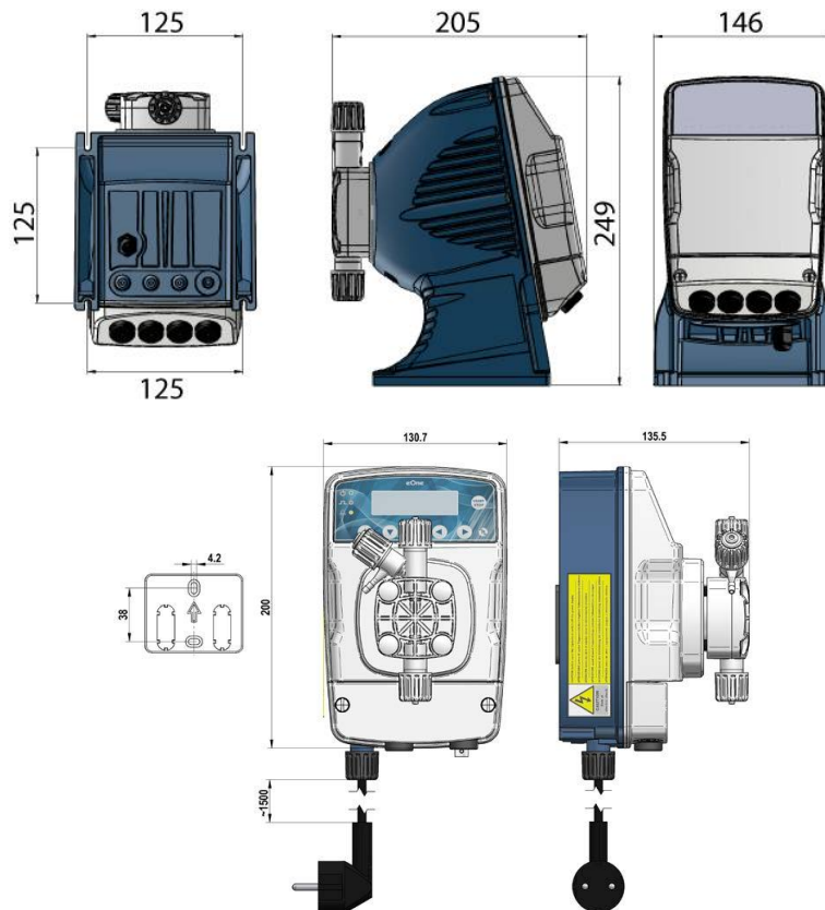
Abb. 1 - Pumpe und Platte für die Wandmontage (Abmessungen in mm)
