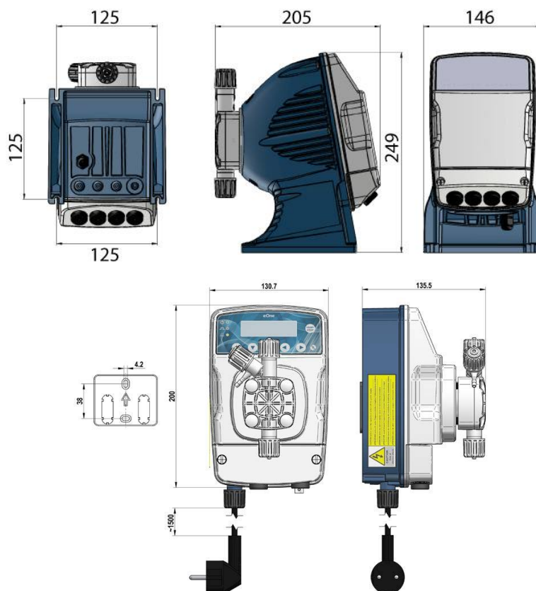
Fig. 1 - Bomba y placa para montaje en pared (dimensiones en mm.)
