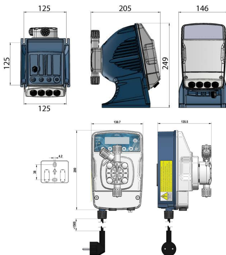
Fig. 1 – Pompa e Placca per il fissaggio a parete (dimensioni indicate in mm.).
