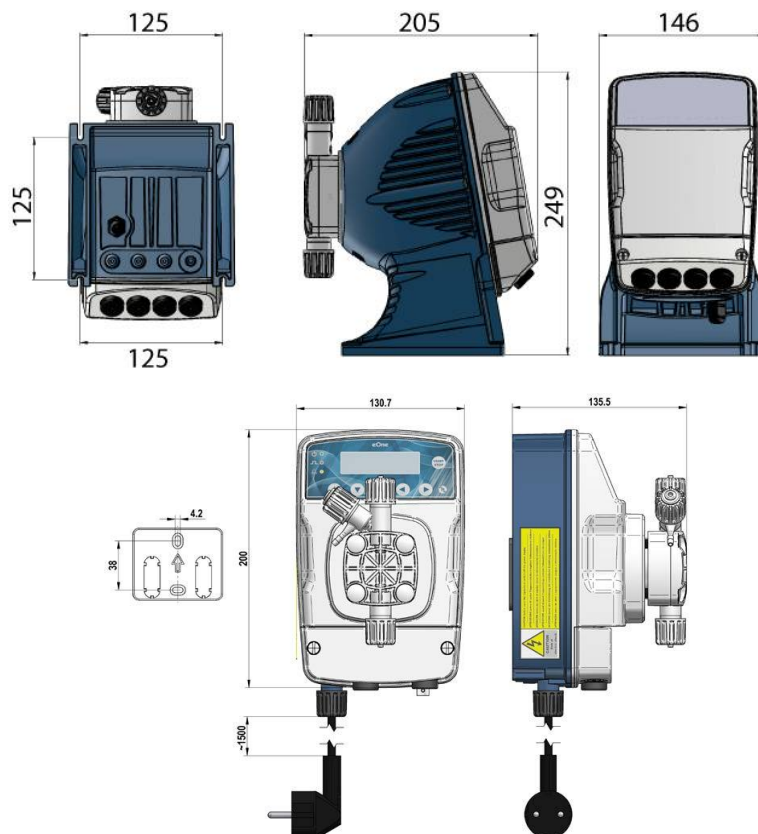
Fig. 1 - Pompe et plaque pour la fixation au mur (dimensions indiquées en mm).
