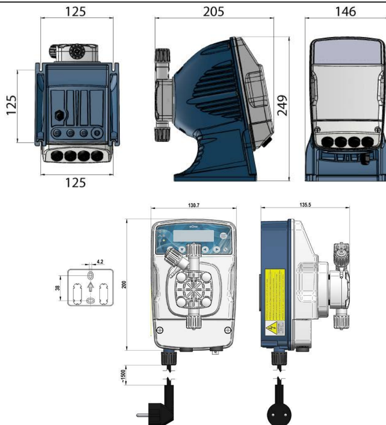
Fig. 1 - Bomba e placa para montagem na parede (dimensões em mm.)
